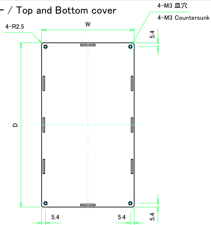
上カバー表面 / Top cover Frontside
