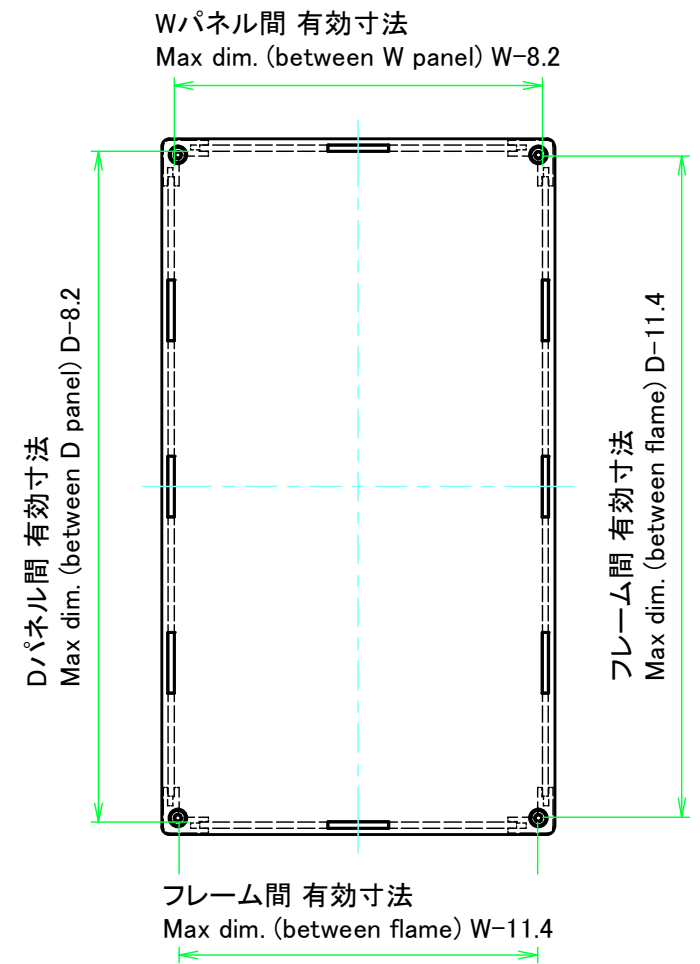
下カバー / Bottom cover
